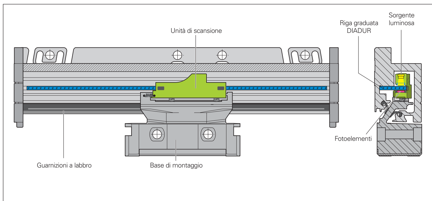
Schema costruttivo del sistema di misura lineare incapsulato LC 183
