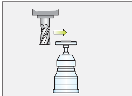
Misurazione raggio utensile
